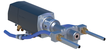
JP5000® HVOF gun
